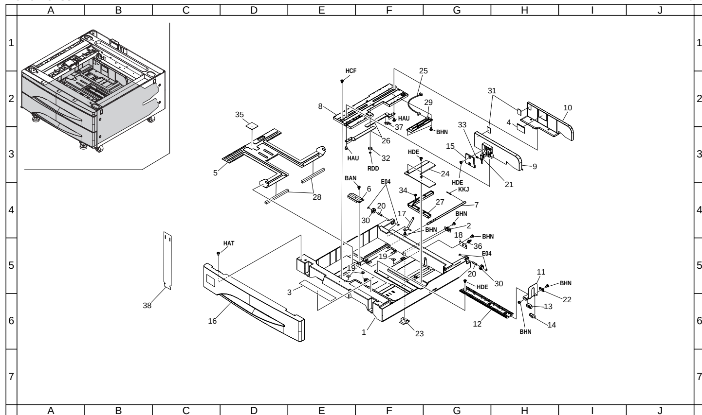
FIG. 3 CASSETTE
