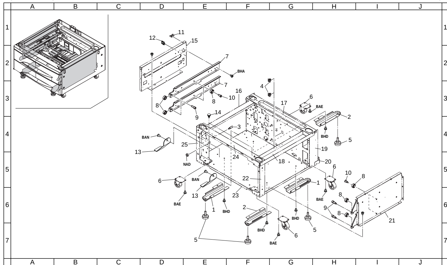
FIG. 2 FRAMES
